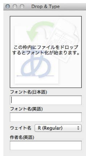
Drop&Type 画面
